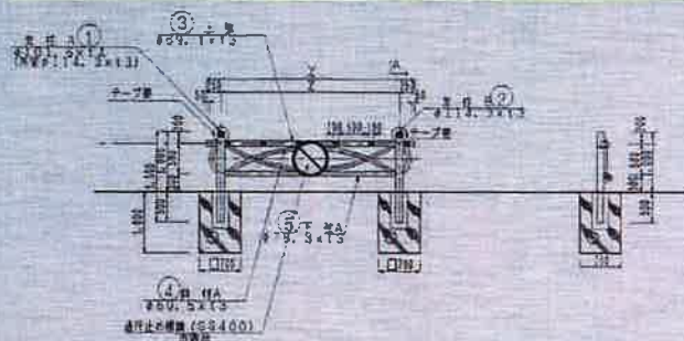
配置詳細図
